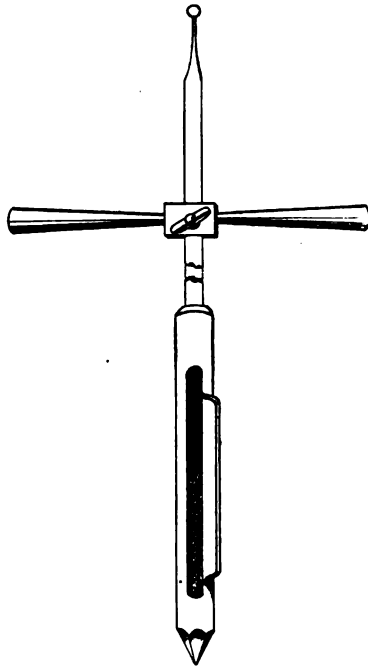
FIG. 218.—Fraenkel's borer.
